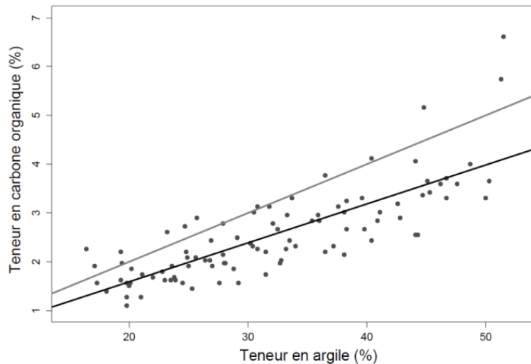
Figure 34 : Relation entre la teneur en argile et le taux de matière organique (Boivin, 2022 ; d'après Johannes et al., 2017)
